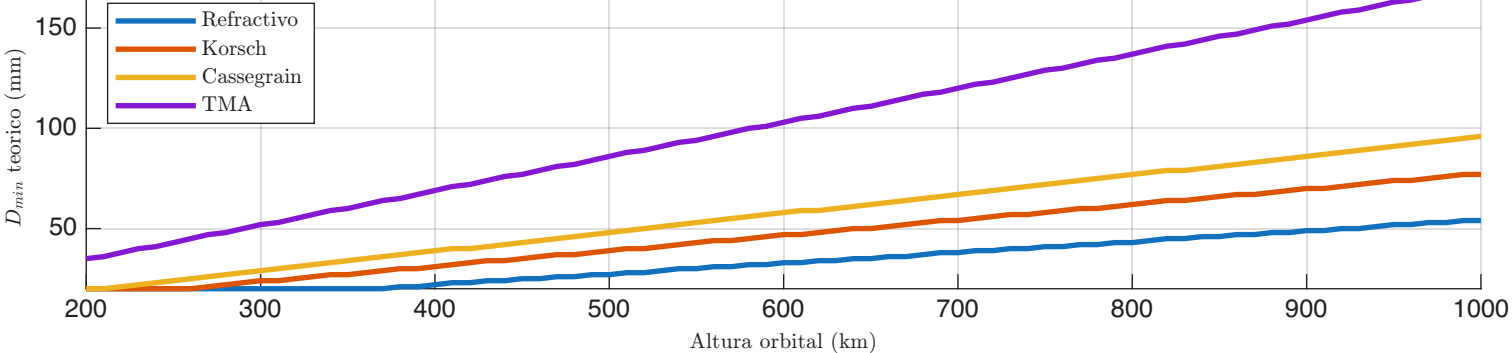
Detector 3: mínimo teórico por MTF/SNR - Configuración: 1 satélite(s), 1 telescopio(s) por satélite
